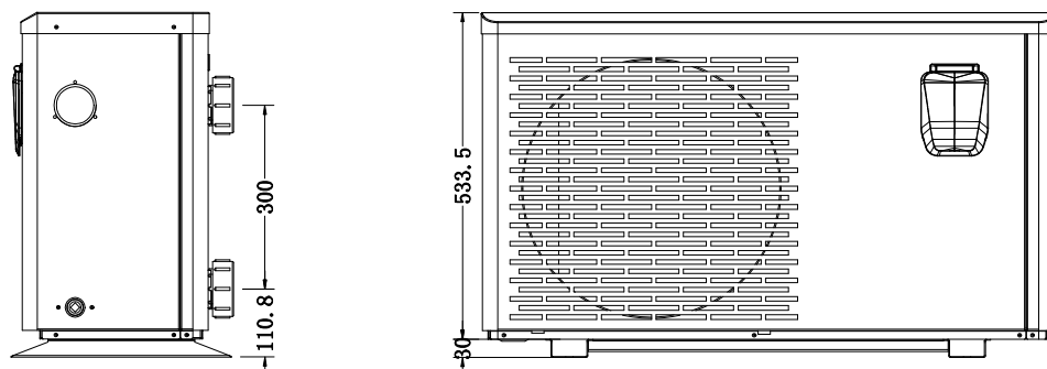
Pompa ciepła 1401
