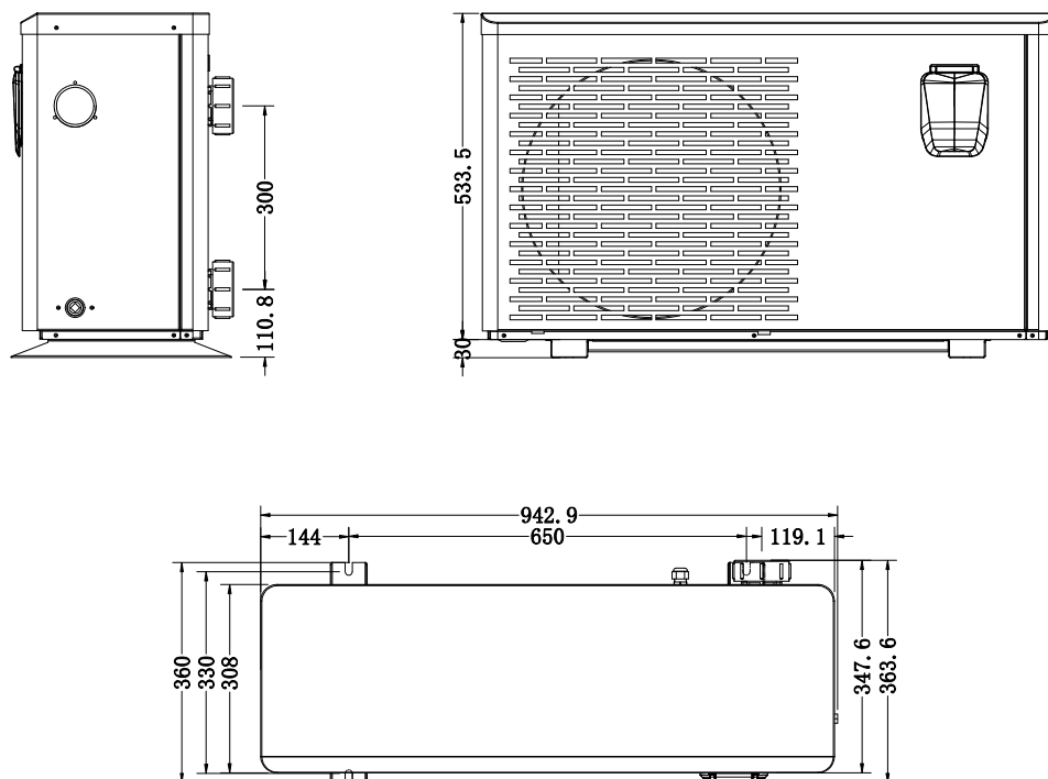
Lämpöpumppu 1402, 1403 ja 1404
