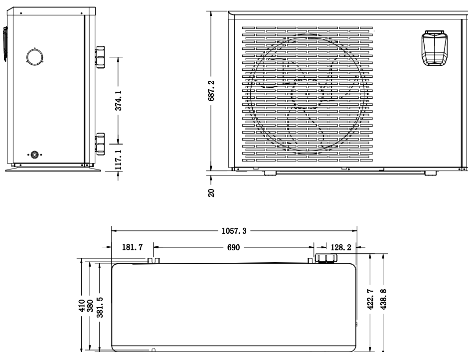
Warmtepomp 1402,1403 en 1404
