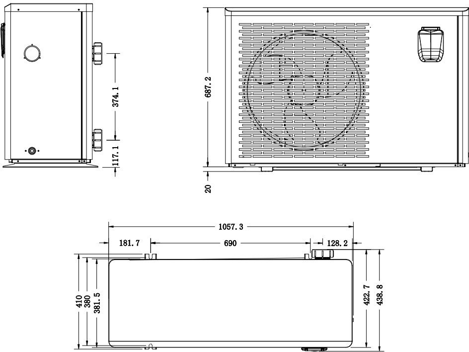
Varmepumpe 1402, 1403 og 1404
